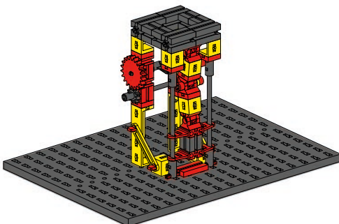
Kniehebelpresse / Toggle press / Presse à genouillère / Kniehefboompers / Pulsar el botón / Alternar a prensa / Premere il pulsante / Тумблерное нажатие / 切换式压力机..... 26
