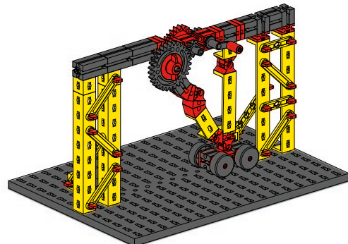
Kniegelenk mit Überstreckung / Knee joint with hyperextension / Articulation du genou avec hyperextension / Kniegewricht met hyperextensie / Articulación de la rodilla con hiperextensión / Joelho articulado com hiperextensão / Articolazione del ginocchio con iperestensione / Коленный сустав при гиперэкстензии / 膝关节伸展器..... 30
