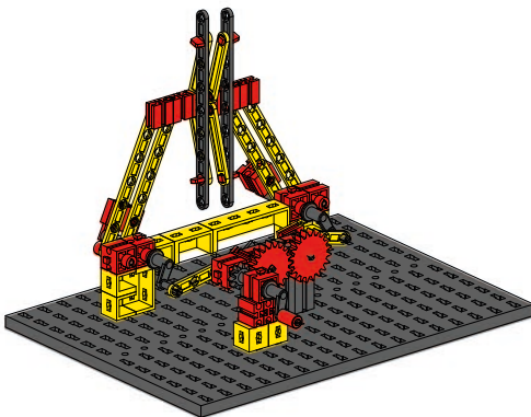
Scheibenwischer - parallel / Windshield wiper - parallel / Essuie-glace - parallèle / Ruitenwissers - parallel / Limpiaparabrisas - paralelo .. / Limpador de pára-brisas - paralelo / Tergicristalli - paralleli / Стеклоочиститель ветрового стекла - параллельно / 平行式雨刮器..... 17
