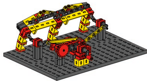
Scheibenwischer - gegenläufig / Windshield wiper - counterrotating / Essuie-glace - à contre-sens / Ruitenwissers - tegengesteld draaiend / Limpiaparabrisas - contra-rotación / Limpador de pára-brisas - contra-rotativo / Tergicristalli - controrotanti / Стеклоочистители ветрового стекла - противовращающиеся / 对刮式雨刮器..... 11
