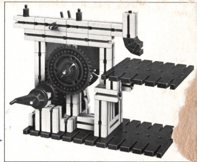
Die Hobelmaschine The planing machine La raboteuse Schaafmaschine
