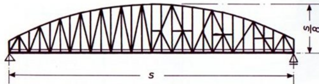
31.4 Halbparabelträger für große Stützweiten (100–200 m), Netzhöhe h etwa 1/8 der Stützweite. Wesentliche Gewichtsverringern durch Verkürzung der Pfosten und Streben nach den Trägerenden zu. (Rechte und linke Trägerhälfte als Beispiel verschieden ausgefächert.)
