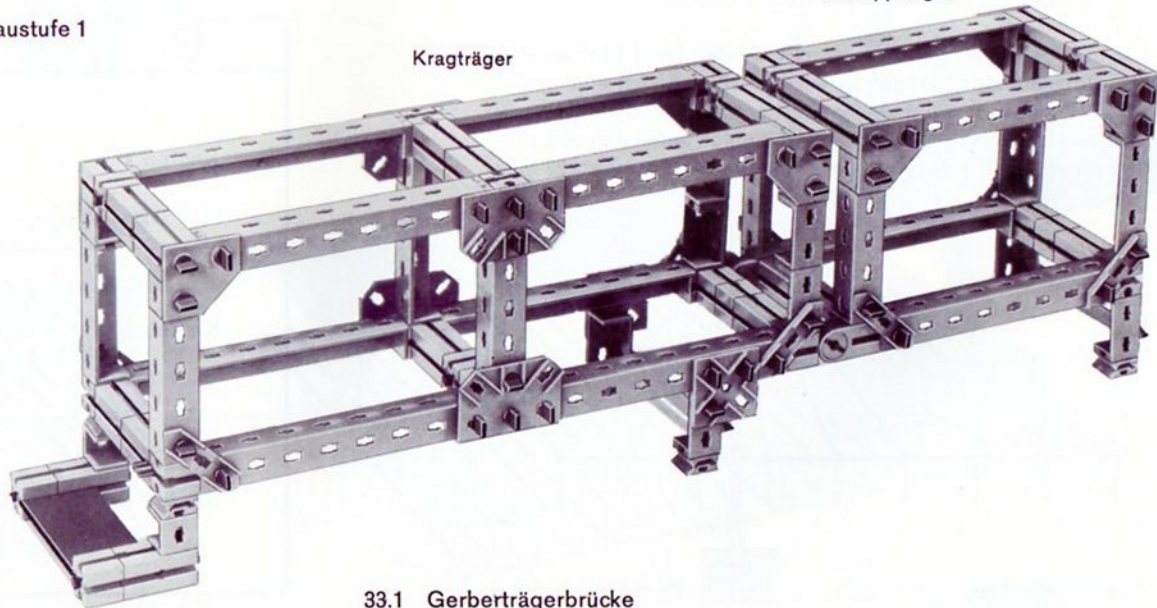
33.1 Gerberträgerbrücke
