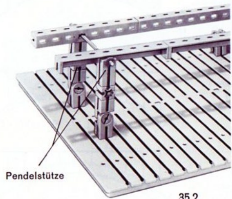
35.2 Baustufe 1
