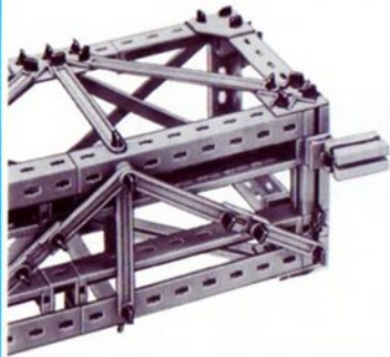
29.5 Fahrbahnträger von unten (Baustufe 1)
