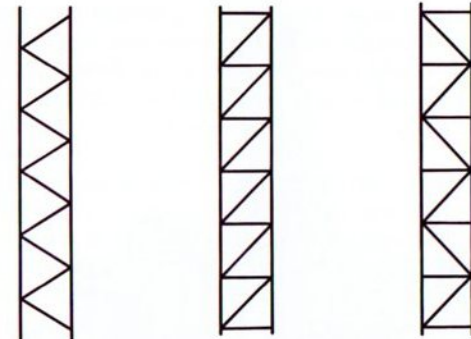
76.1 Gittermaste
