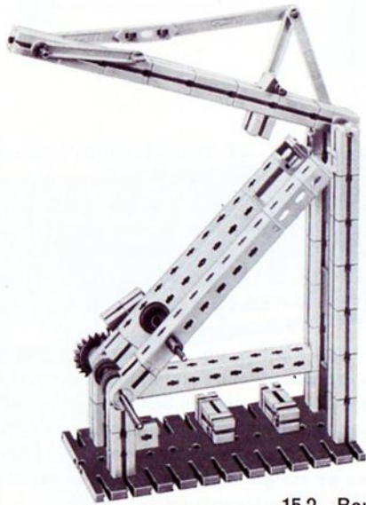
15.2 Baustufe 1
