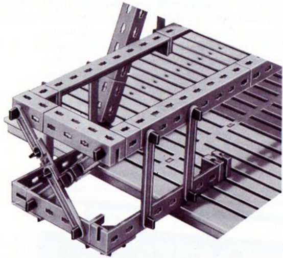
40.2 Brückenpfeiler rechts, Rückseite
