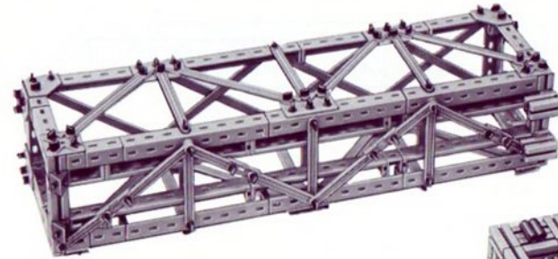
29.3 Fahrbahnträger von unten
