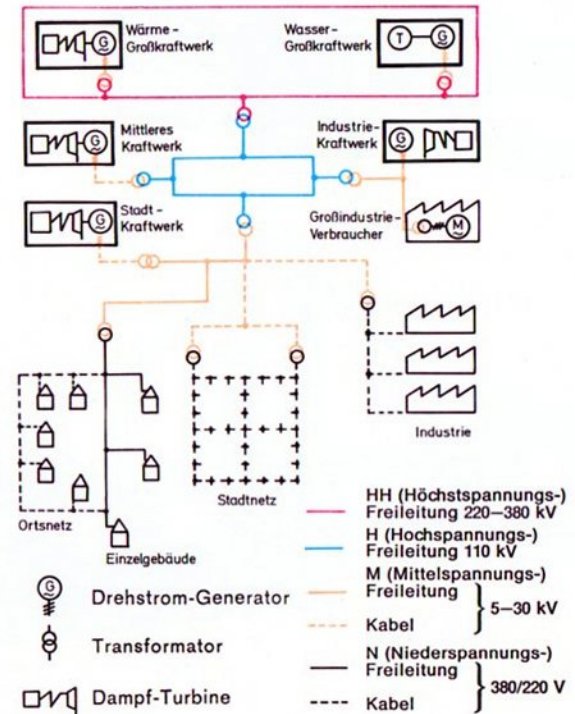
48.1 Energie-Verteilung
