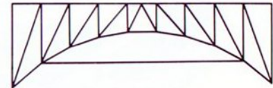
24.8 Zweigelenkbogen mit Zugband (einfach inner- lich statisch unbestimmt)
