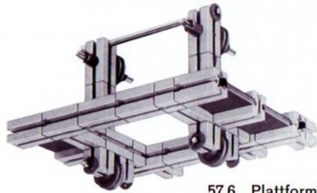
57.6 Plattform von unten
