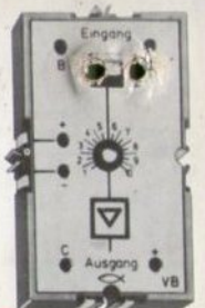
1 Verstärker-Baustein
